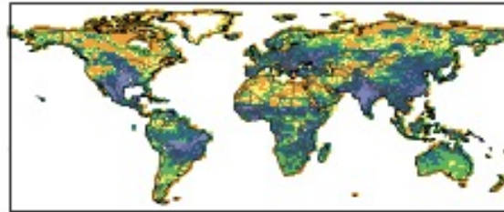
JJA
