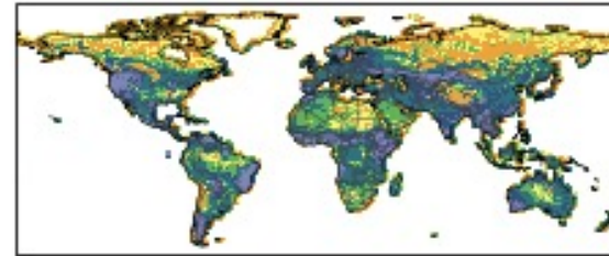
MAM
