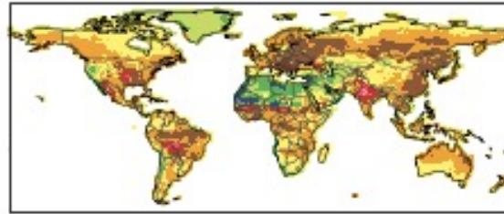
JJA
