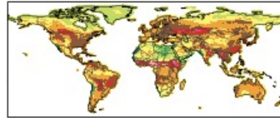
MAM
