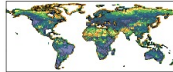
SON
