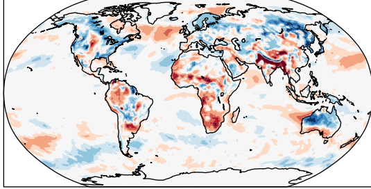
SON PBLH Daily 12
